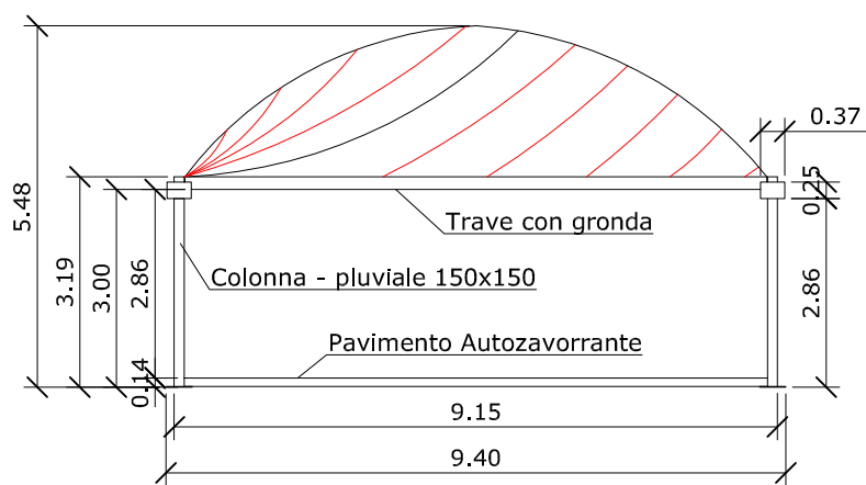
- PROSPETTO
