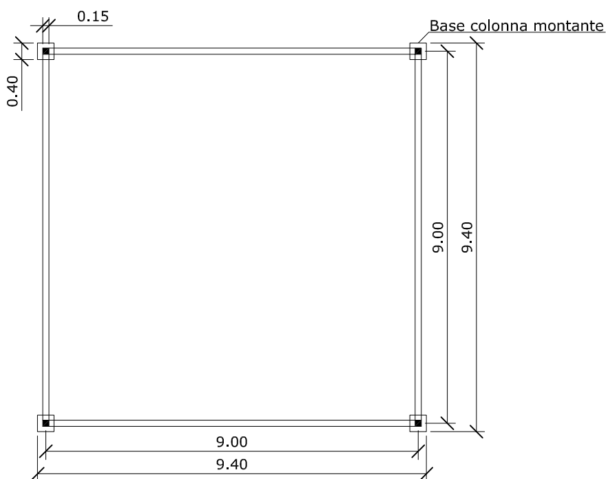
- PIANTA
